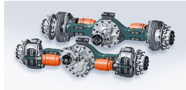
Leichtes Hypoidachst tandem
