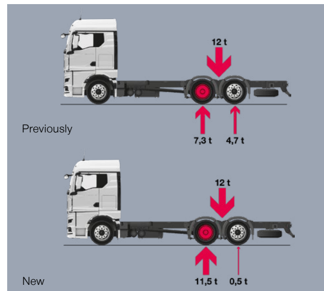
Variables Achslastverhältnis
