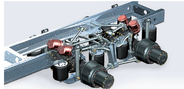
Bauluftfederung
