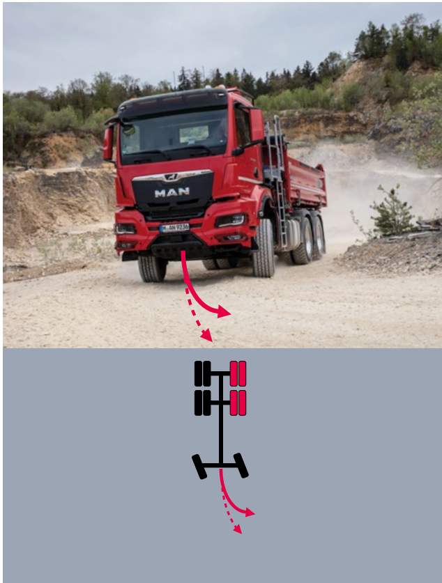
Funktionsprinzip Lenkbremse
